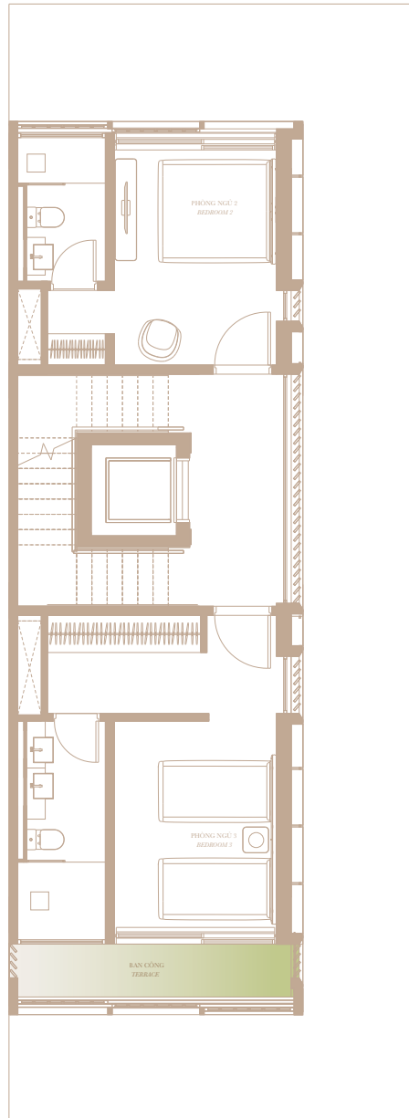
LẦU 3 Level 3
