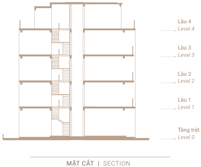
MẶT CẮT | SECTION
